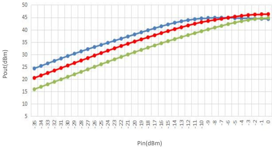
Pout@Pin
