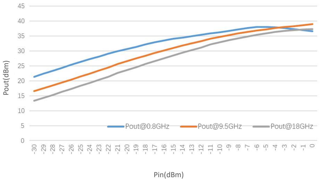
Pout@Pin
