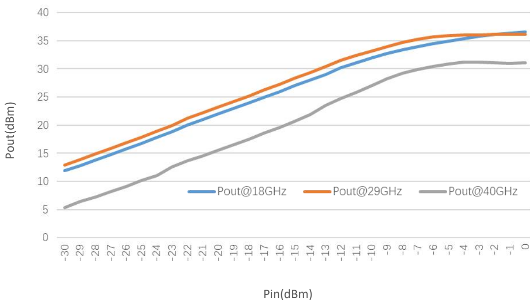
Pout@Pin
