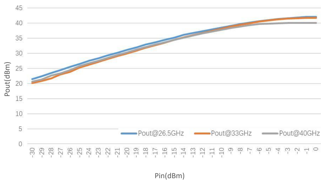
Pout@Pin
